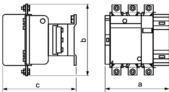
Рисунок 8. Контактор LC1E200...300
