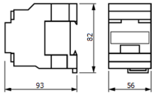
Рисунок 3. Контакторы LC1E25
