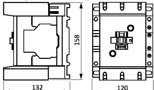
Рисунок 7. Контакторы LC1E120...160
