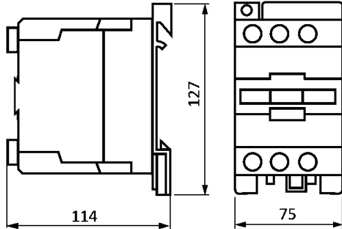
Рисунок 5. Контакторы LC1E40...65
