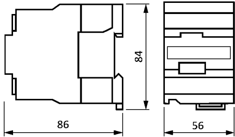
Рисунок 2. Контакторы LC1E06...18
