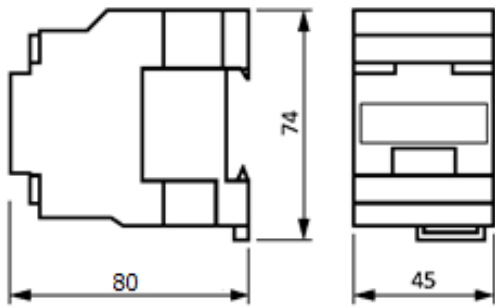
Рисунок 2. Контакторы LC1E06...18
