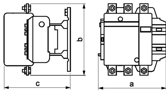
Рисунок 9. Контакторы LC1E400...500
